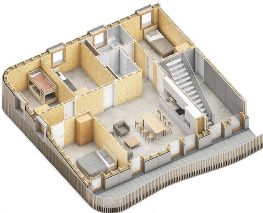
6 Isometrie einer Wohnung im Hoffnungshaus Flandernstraße
